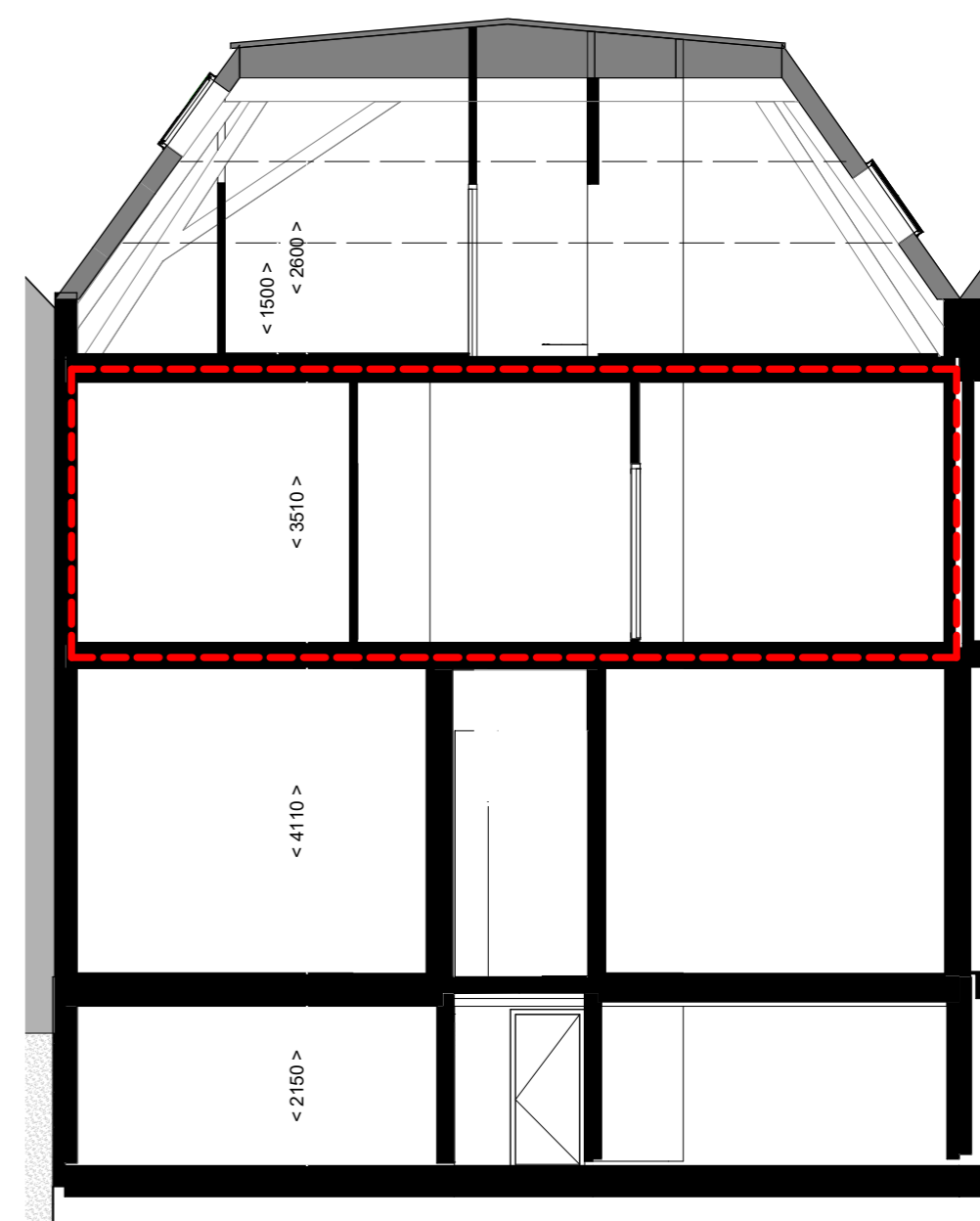
doorsnede N11b
