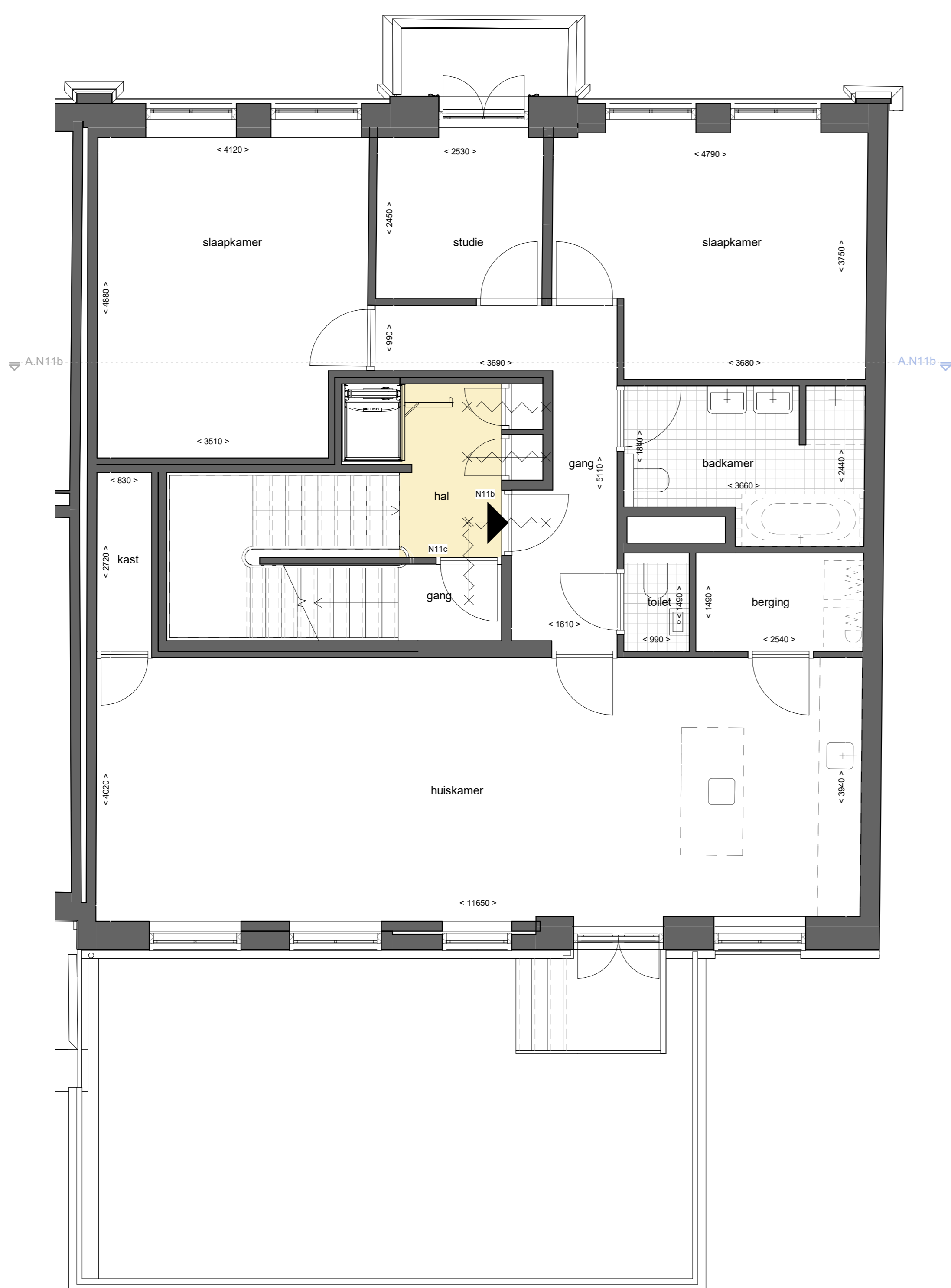
eerste verdieping
