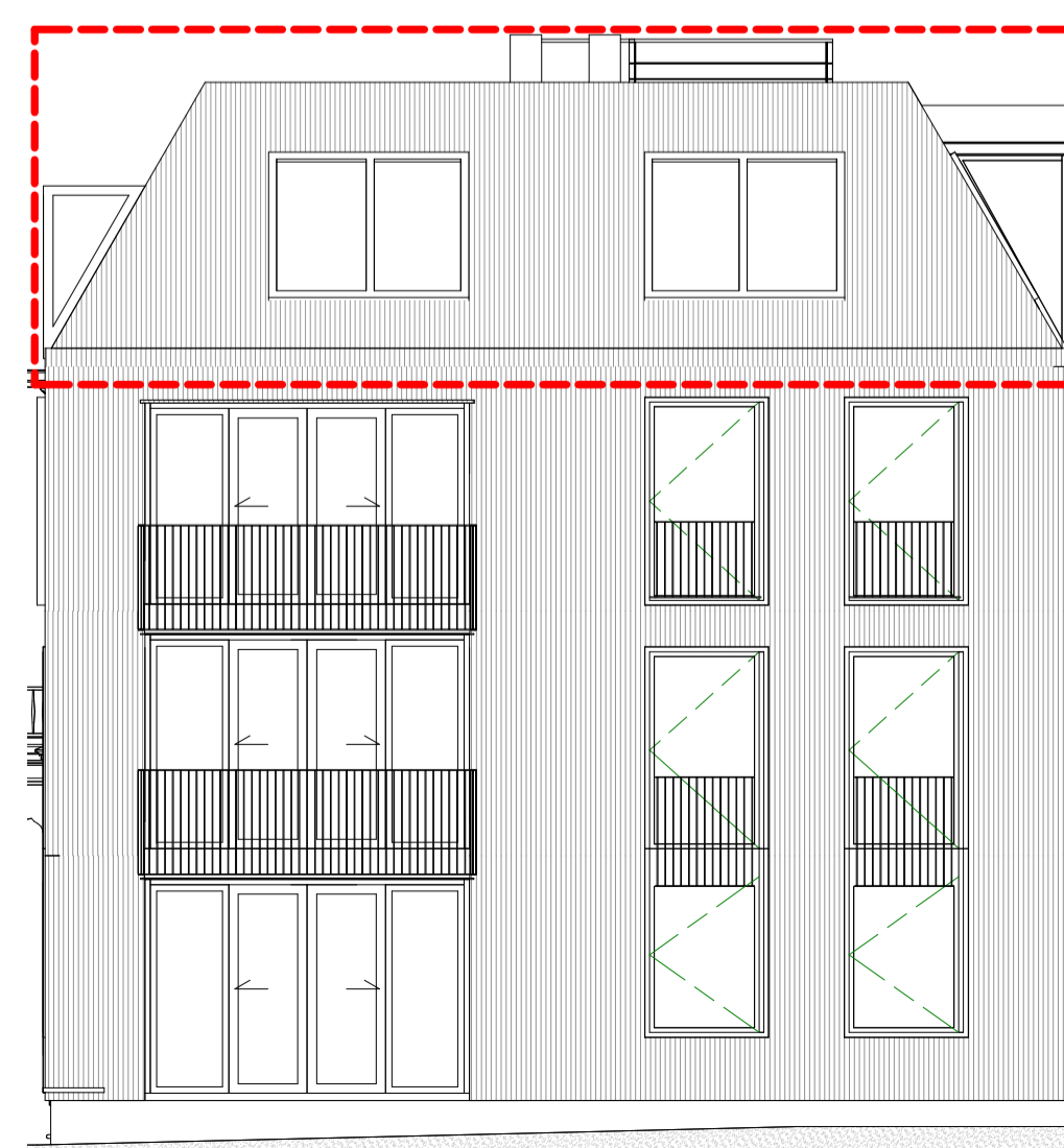
kopgevel Kapjeswelle
