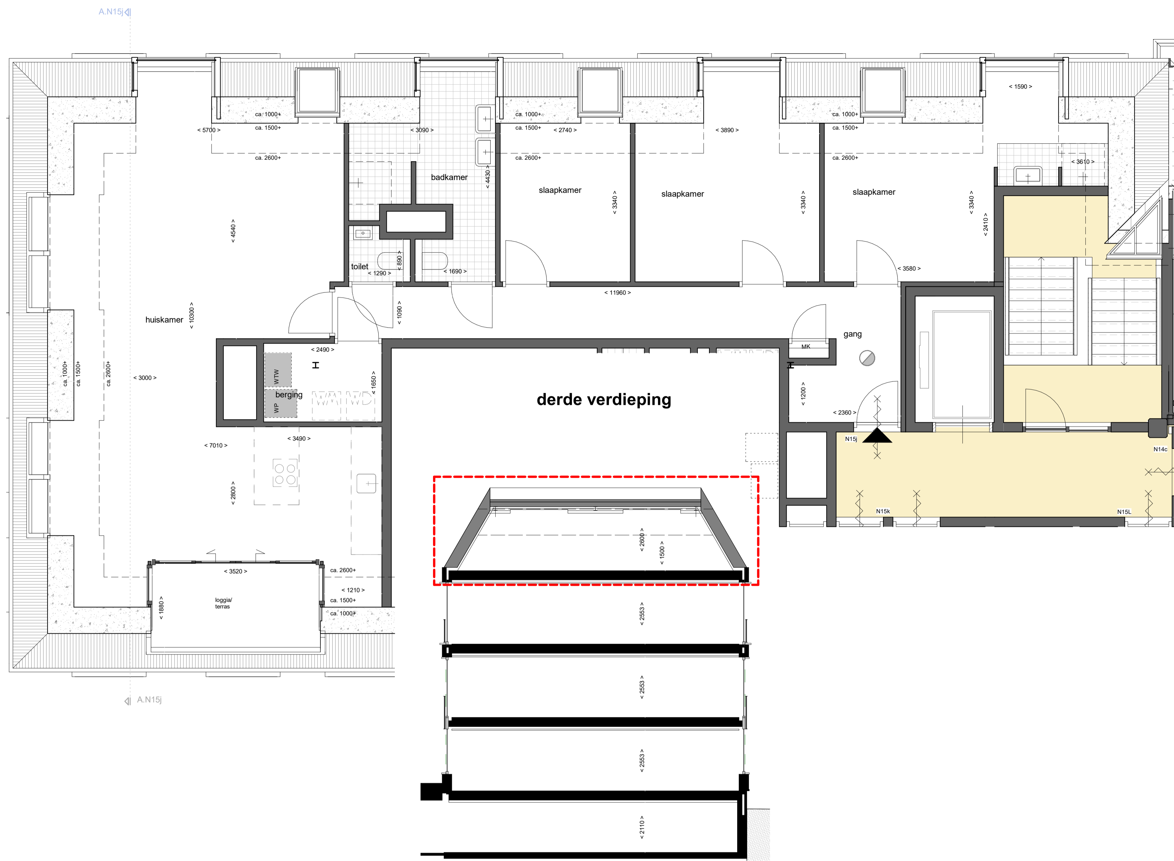
doorsnede N15j
