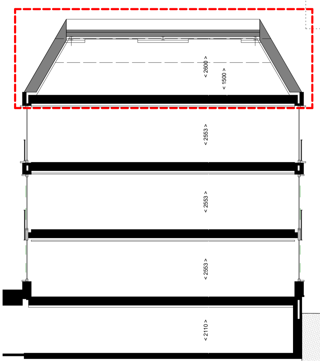
doorsnede N15j
