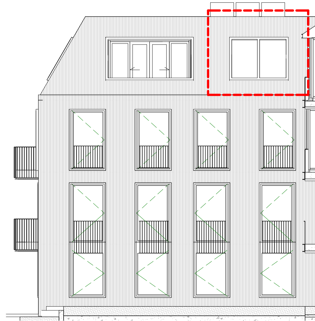
zijgevel Kapjeswelle
