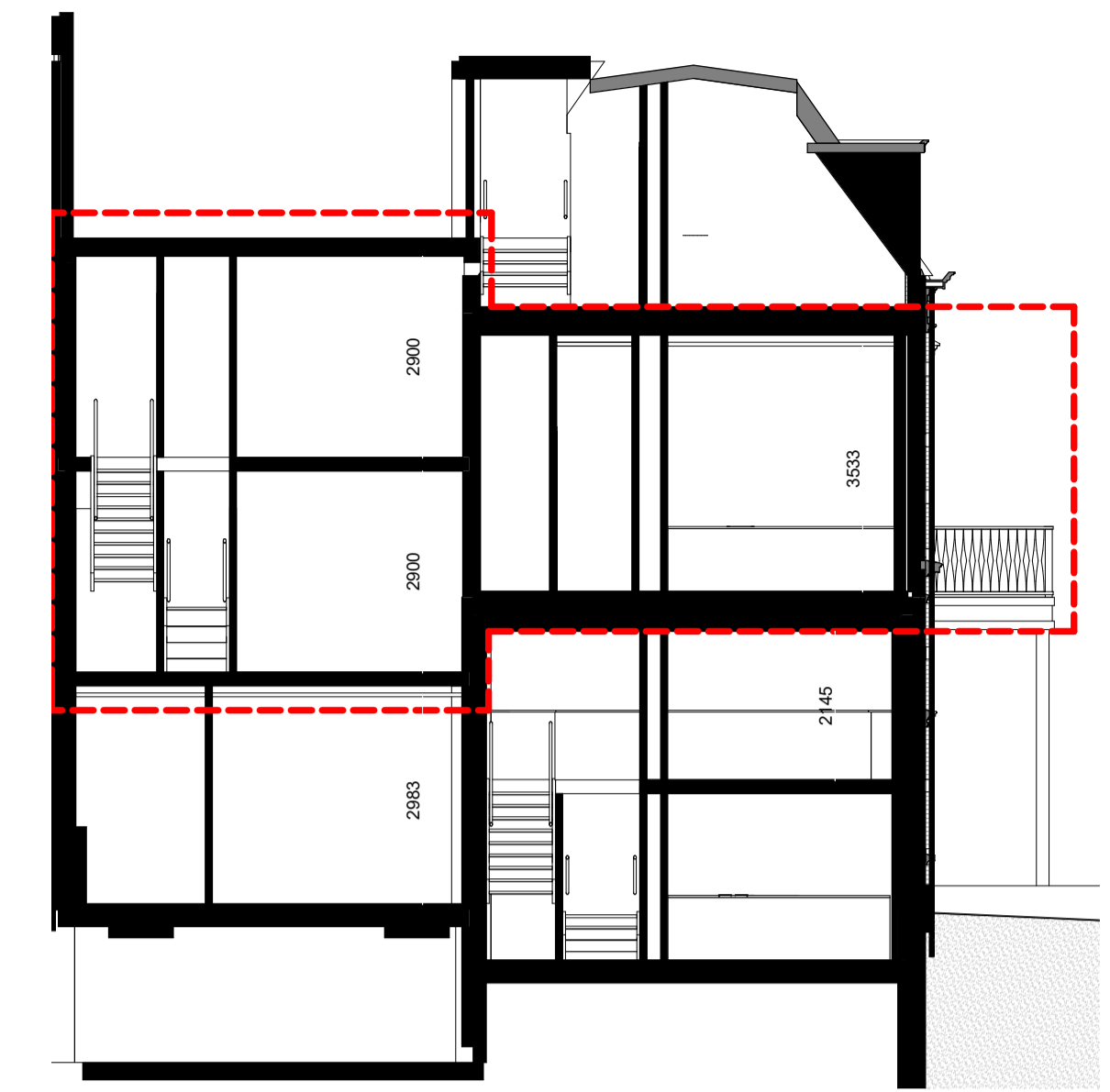
doorsnede T2d2
