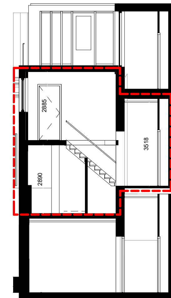
doorsnede T2d1
